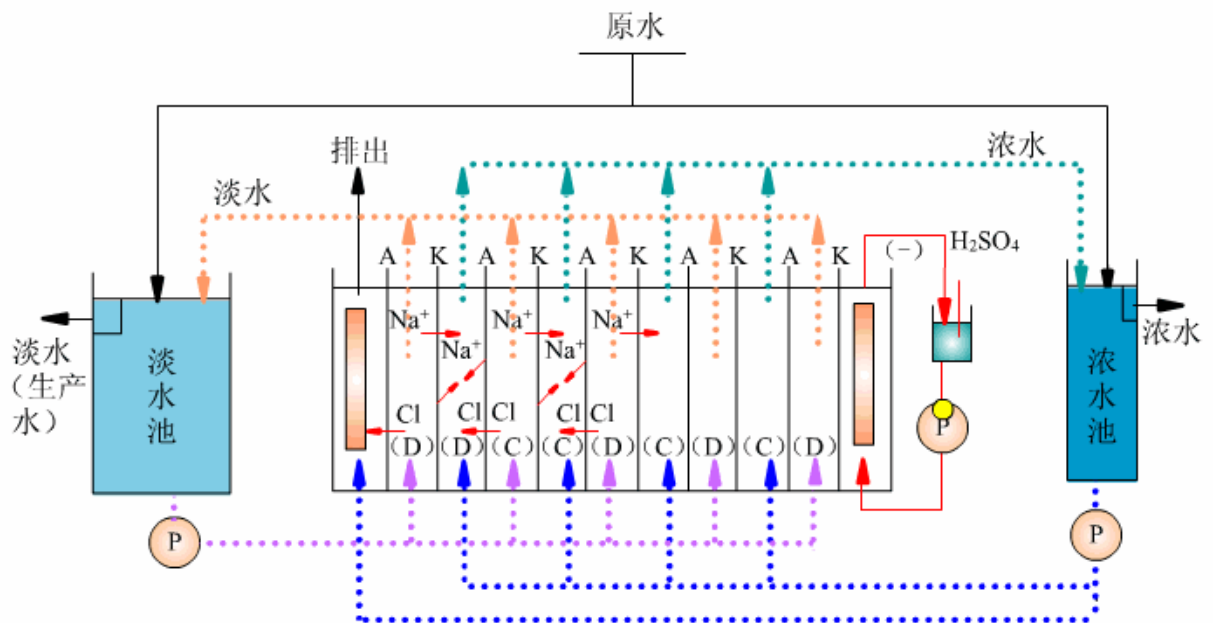
K—阳离子交换膜；A—阴离子交换膜；D—淡水室；C—浓水室
